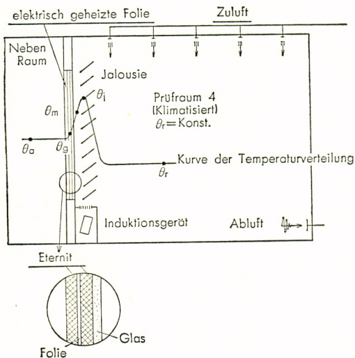
Bild-7 Prinzipieller Aufbau der Versuchsanordnung
