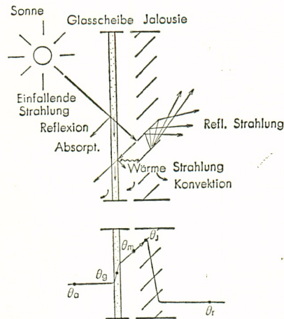
Bild-6 Temperaturverteilung eines klimatisierten Raumes mit halbgeöffneter Innenjalousie für konstante Raum- und Außenlufttemperatur
