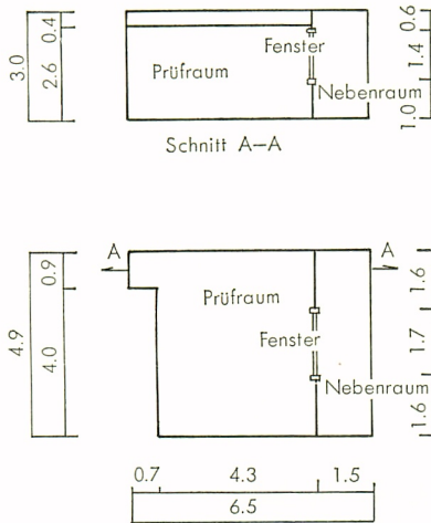
Bild-9 Grundriß des Prüfraumes
