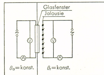
Bild-8 Prinzipielle Aufbau der Versuchsanordnung
