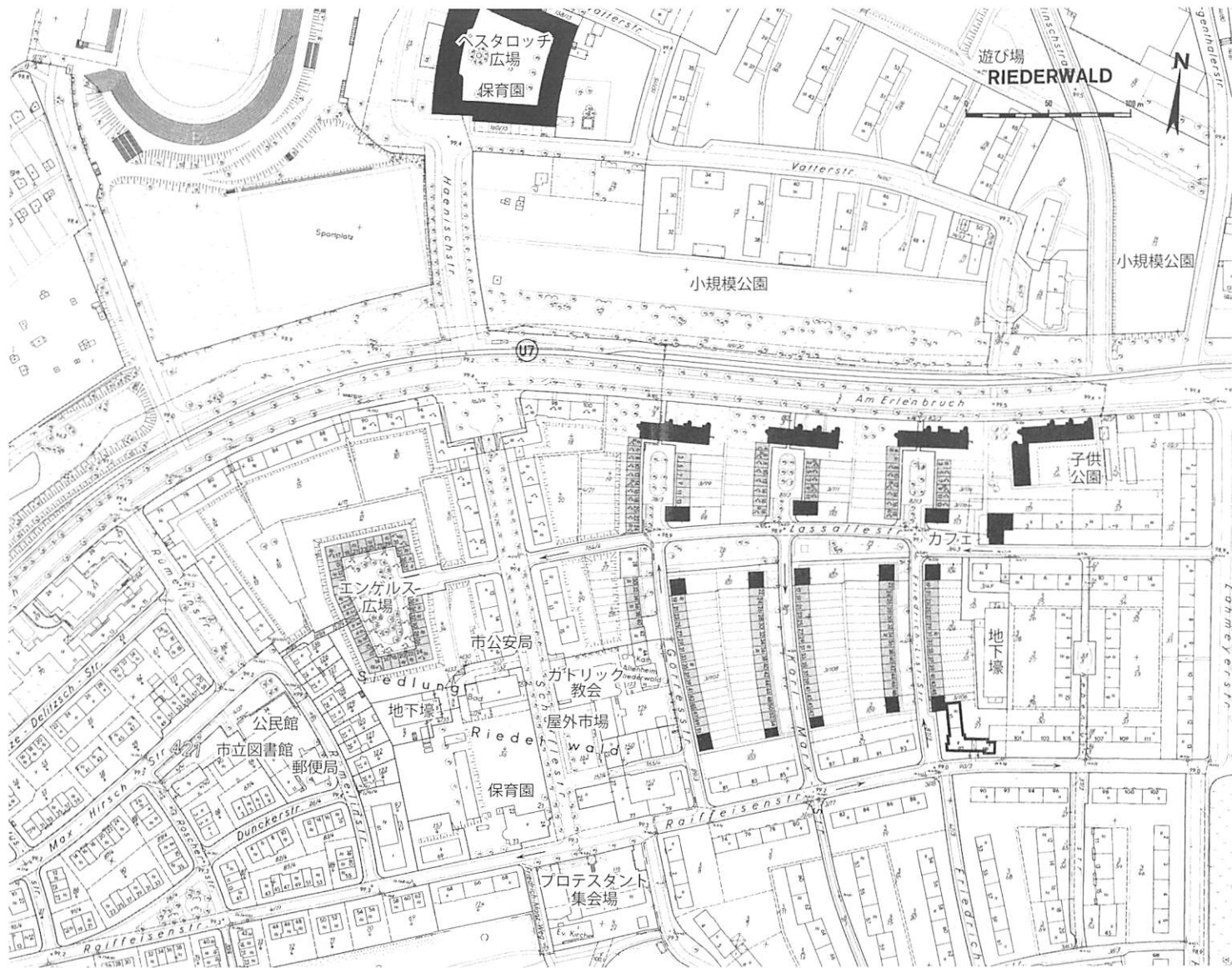
図7 リーダーヴァルトゾーディング敷地配置図(文献5)
