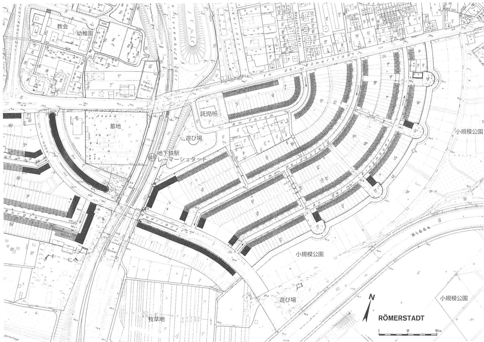
図5 レーマーシュタットジードルング敷地配置図(東部分)文献5)
