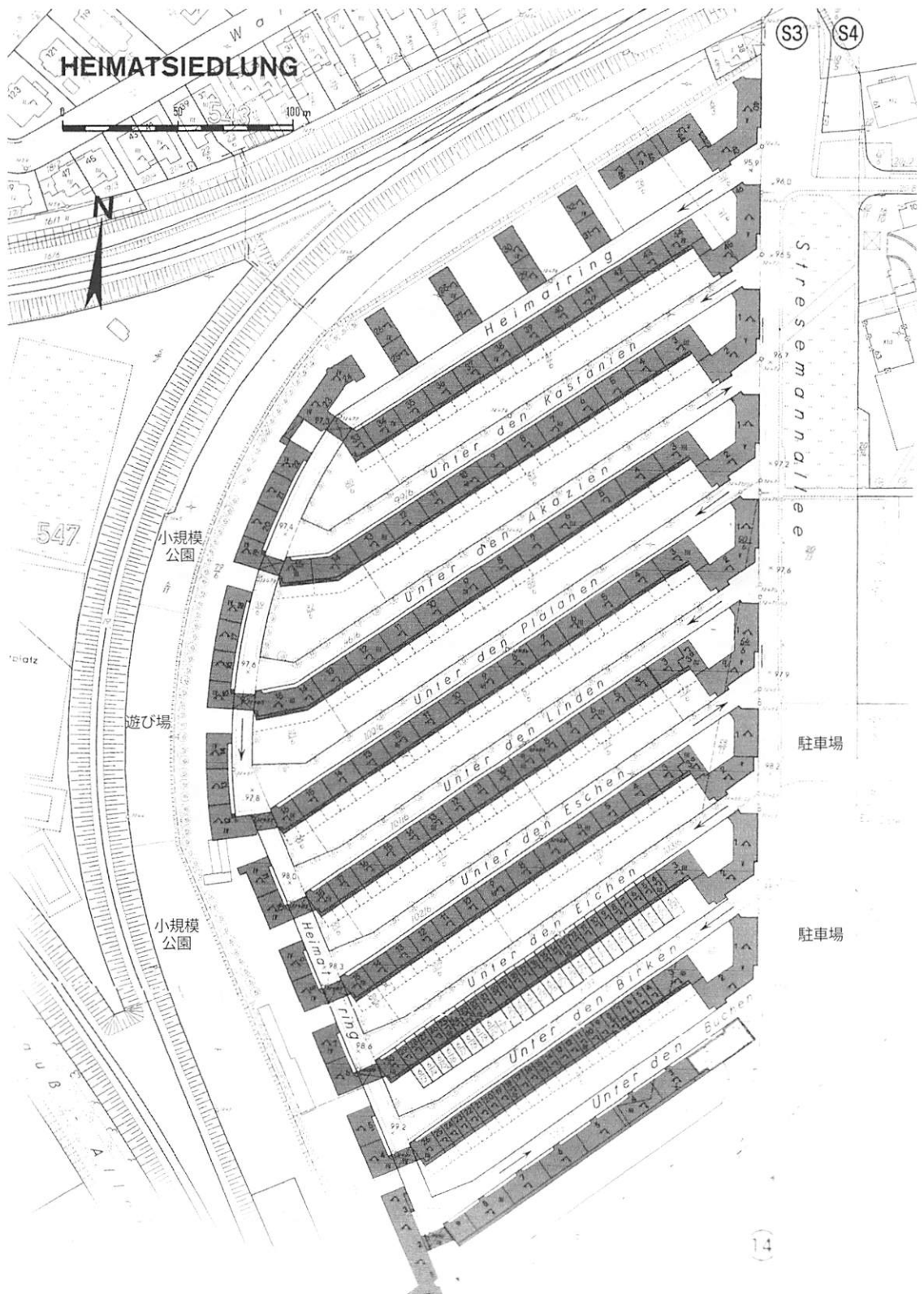
図9 ハイマートジードルング敷地配置図(文献5)
