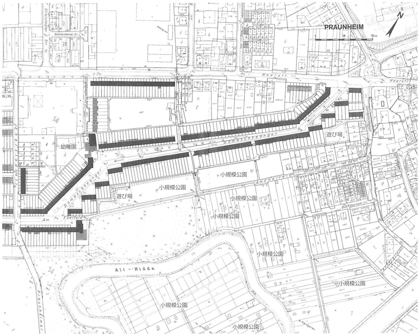
図3 ブラウンハイムジードルング敷地配置図(東部分)文献5)
