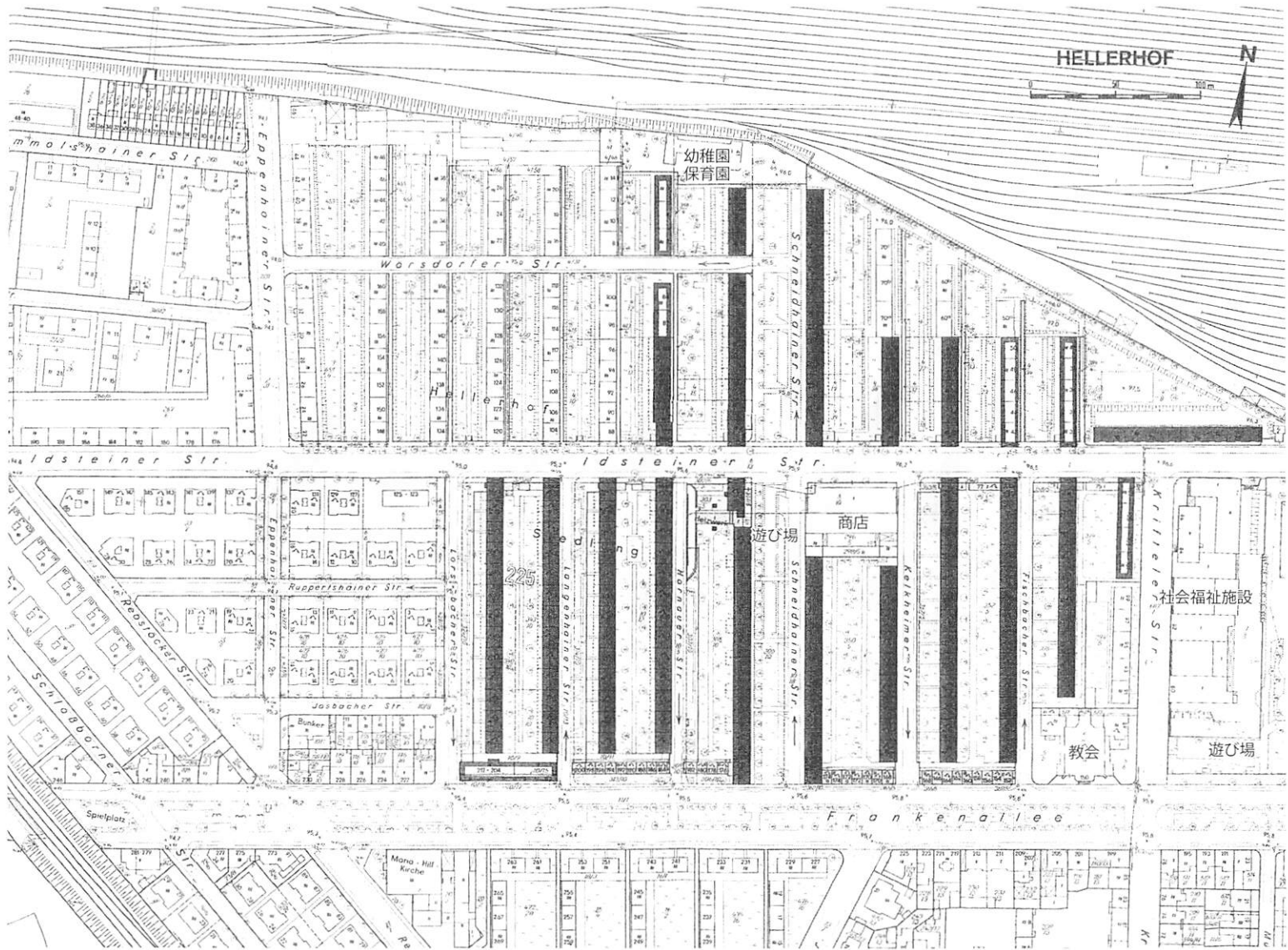
図8 ヘラーホーフジードルング敷地配置図(文献5)
