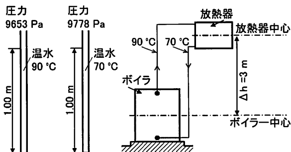
図-10 重力式循環温水暖房の原理
