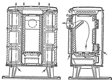
Transportabler keramischer Dauerbrandofen mit Deckenzug und Umluftkanälen
